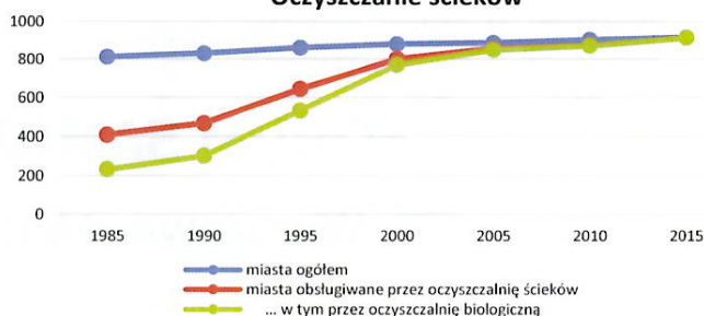
Oczyszczanie ścieków
